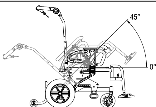
☆ STD tilt (0 → 45°)
